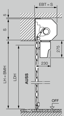
Domaine dimensionnel des portes de garage à enroulement intérieur et extérieur
