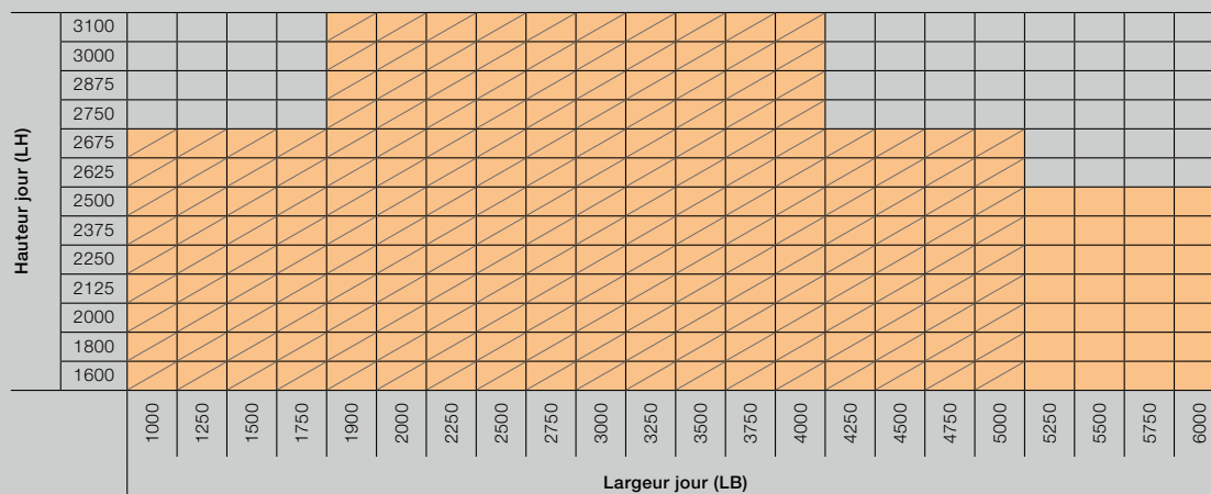
Domaine dimensionnel des portes de garage à enroulement intérieur et extérieur
